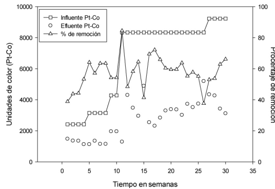
Figura 5. Resultados de la remoción de Color.
