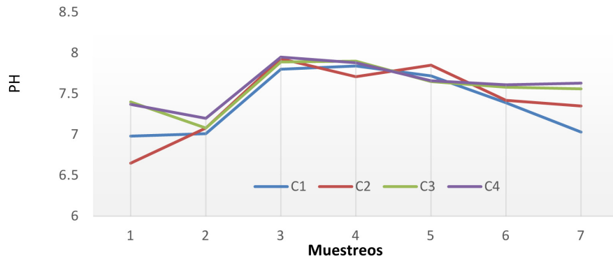
Figura 6. pH registrado en el proceso de biorremediación.
