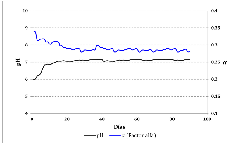
Figura 2. Parámetros de Control del UASB
