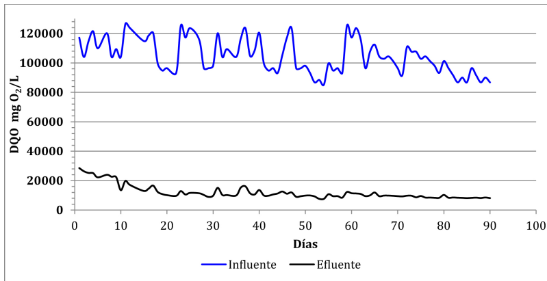
Figura 3. Evaluación del biorreactor UASB.
