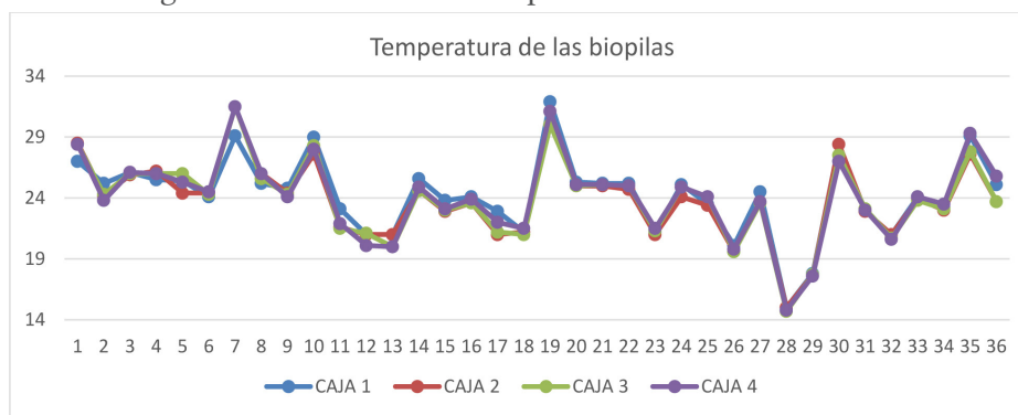
Figura 1. Monitoreo de temperatura en el tratamiento
