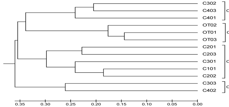
Figura 2. Cladograma del algoritmo UPGMA programa MEGA a través de p-distance. El número en los nodos corresponde a los valores de soporte bootstrap con 100 repeticiones.
